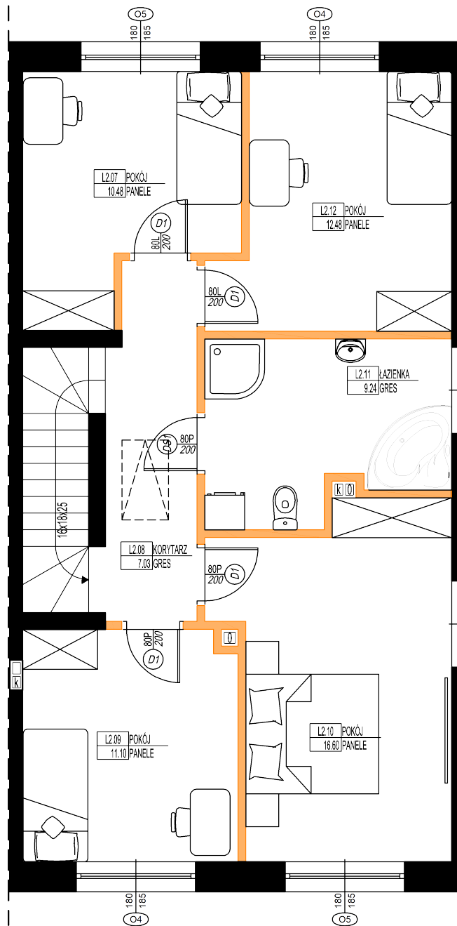
RZUT PIĘTRA
