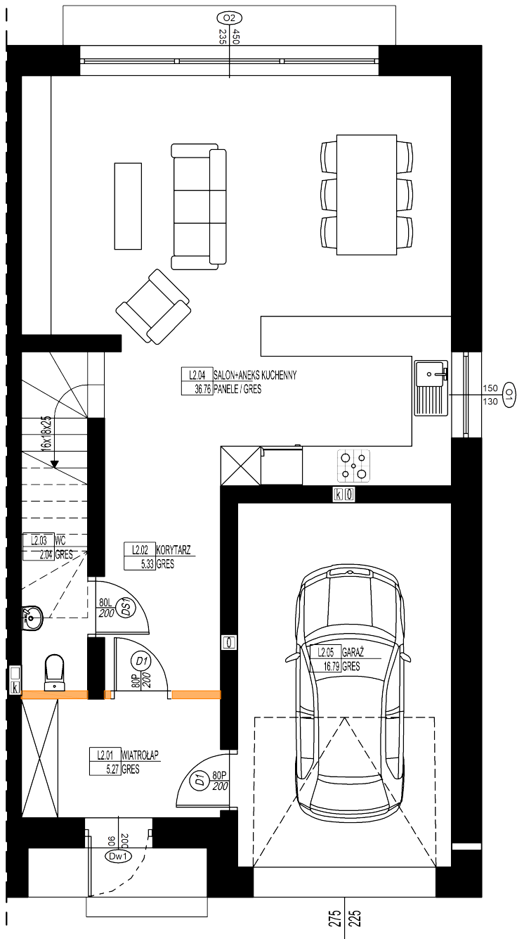
RZUT PARTERU
